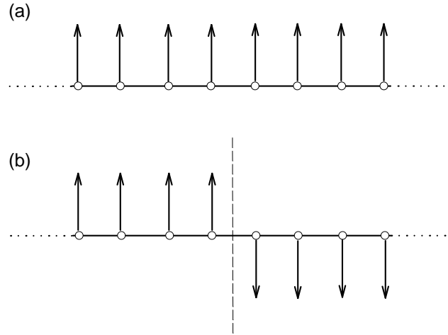
Figura 12: (a) Estado fundamental del modelo de Ising unidimensional. (b) Pared de dominio.
