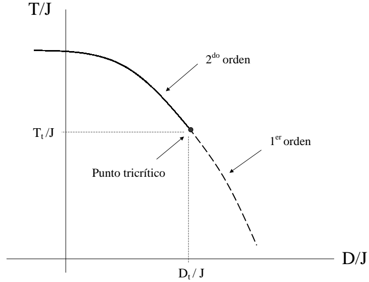
Figura 9: Diagrama de fases esquemático del modelo de Blume-Capel.
