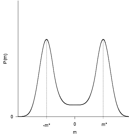
Figura 39: Distribución de probabilidad para la magnetización cuando T < T_c en un sistema finito.
