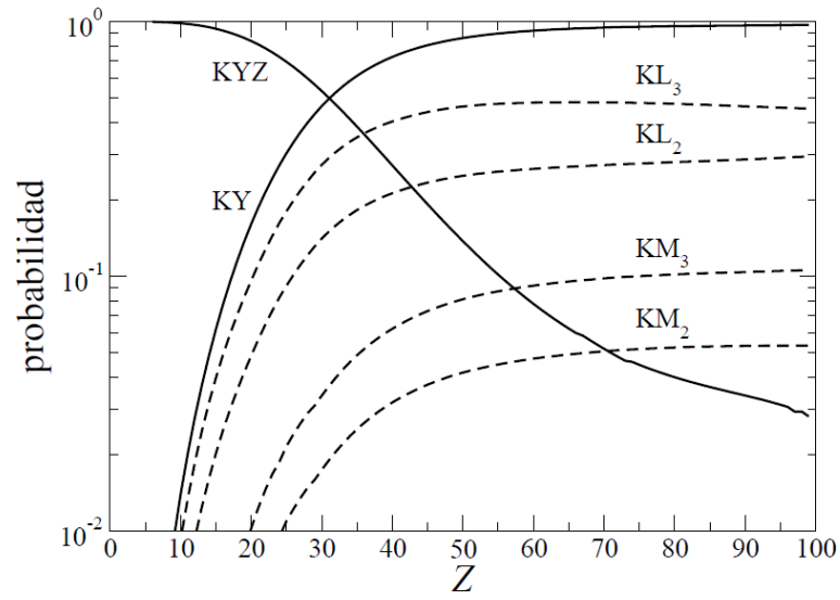
Figura 24. Las curvas continuas representan las probabilidades de las transiciones no radiativas ( KYZ ) y radiativas ( KY ) consecuencia de una vacancia en la capa K , mientras que las curvas a trazos indican las transiciones radiativas más probables ( KL_2 , KL_3 , KM_2 y KM_3 ).
