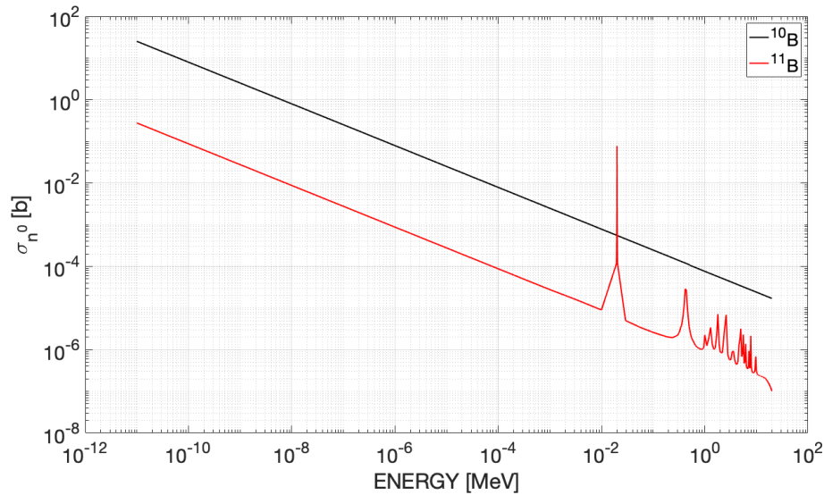
Figura 29. Sección eficaz de para neutrones en {}^{10}\text{B} (rojo) y {}^{11}\text{B} (negro) [IAEA database].
