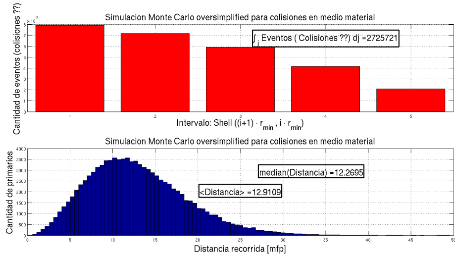
Figura 38. Random walk : Alcance de partículas de emisión por simulación en shells por partículas emitidas en origen de modo isotrópico en un medio homogéneo.
