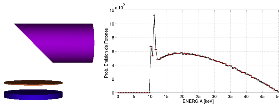
Figura 47. Espectro de emisión de tubo de rayos X de ánodo de W irradiado con electrones de 50 keV (filtro de Al) obtenido con PENELOPE.
