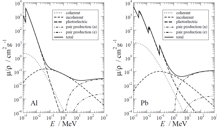
Figura 9. Coeficientes de atenuación másicos de Al y Pb, obtenidos con el programa XCOM.
