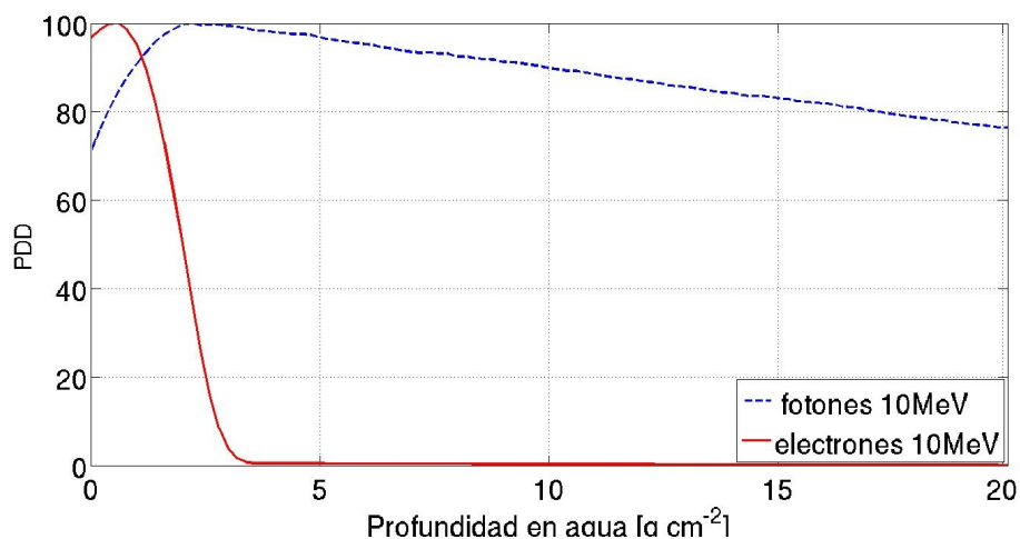
Figura 27. Porcentaje de dosis en profundidad para un haz de 10MeV de fotones (azul) y de electrones (rojo) en agua obtenido con FLUKA bajo licencia de código de usuario FUID-2038 de FLUKA Collaboration CERN.
