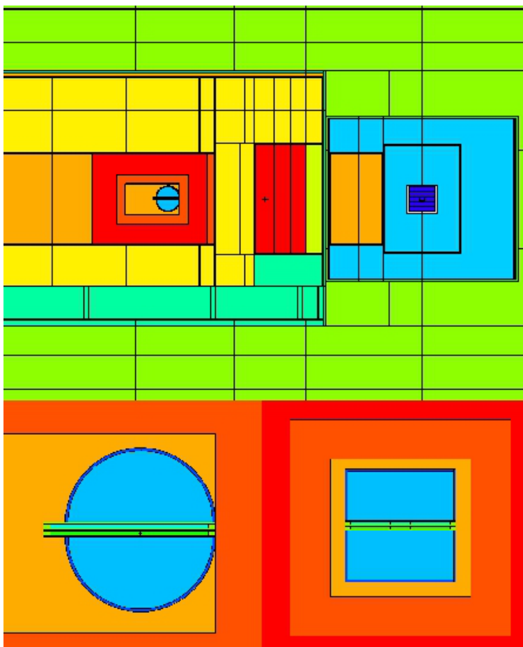
Figura 31. Esquema del reactor, core y columna con disposición de fantasmas y dosímetros.
