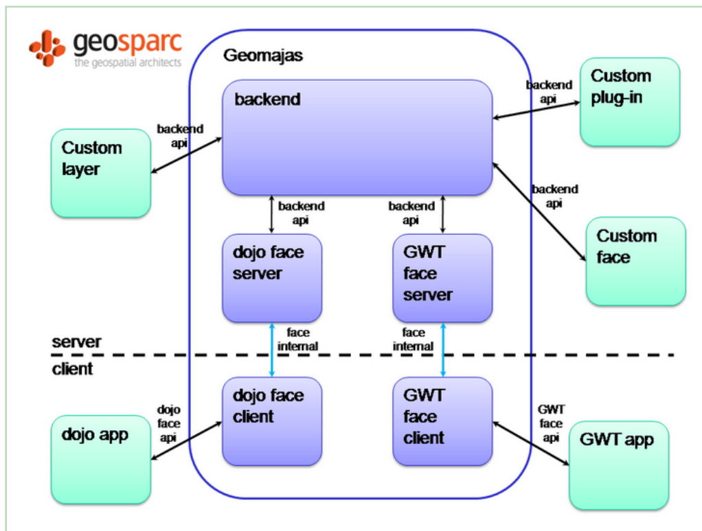
Figura 4.4: Arquitectura de Geomajas, extraído de: Geomajas user guide for developers, capítulo Architecture
