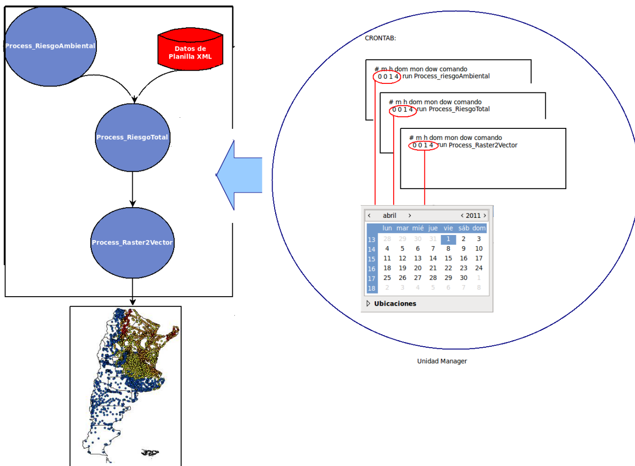
Figura 5.5: Proceso completo y ejecución de los mismos por la unidad manager
