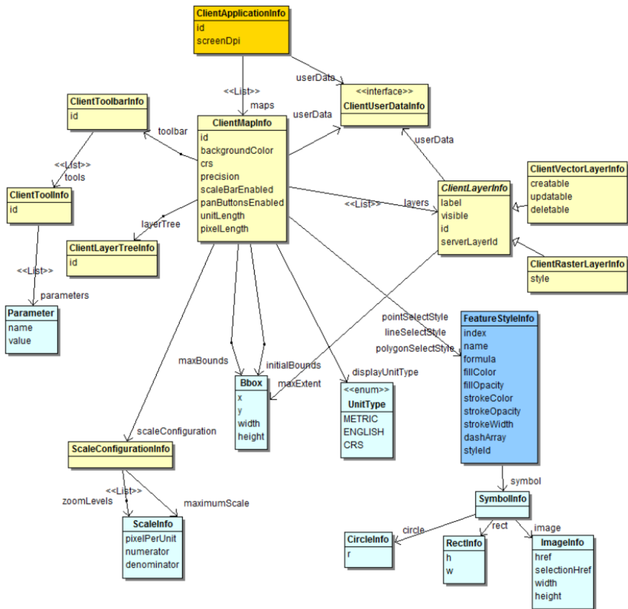
Figura 5.18: Resumen de los Objetos a Configurar en la unidad GIS Web Viewer
