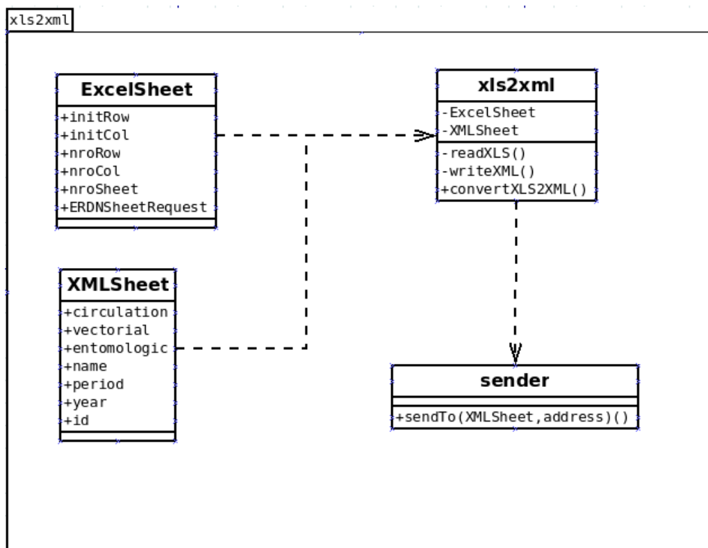
Figura 5.2: Diseño Técnico de la unidad xls2xml
