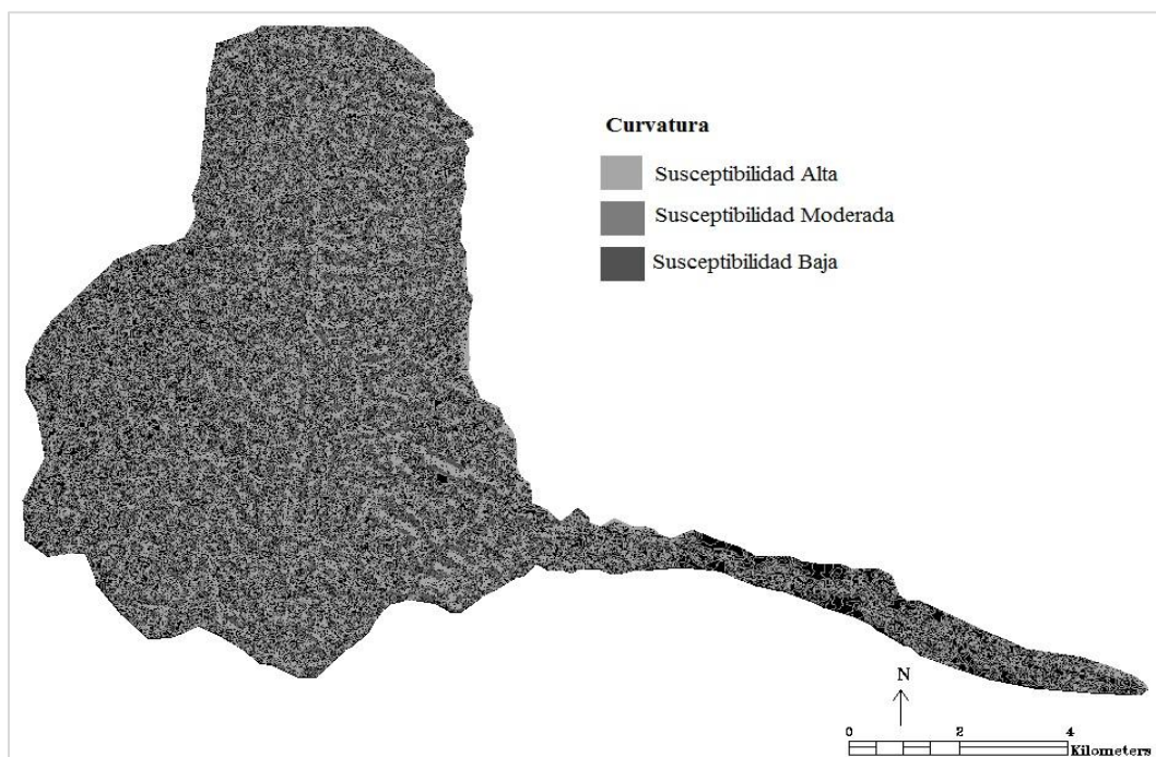
Figura 35. Mapa de Susceptibilidad del terreno debido a la curvatura.
