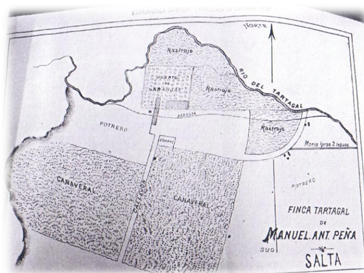
Figura 17. Mapa de la antigua Finca Tartagal, Salta (Argentina) (Alonso, 2012).
