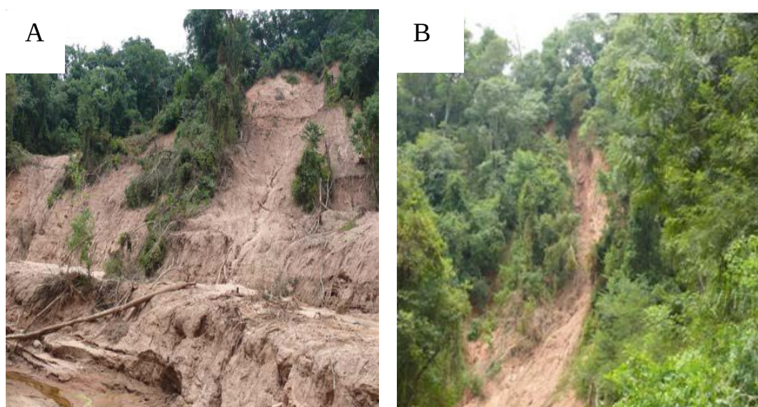
Figura 23. Quebrada del Aguay en la cuenca alta del río Tartagal. A) Se observa erosión en el cauce principal, movimientos de masa en las laderas y depósitos de troncos, ramas y sedimentos que dejaron los flujos a su paso; B) Avalancha de detritos (Baumann et al. , 2009).
