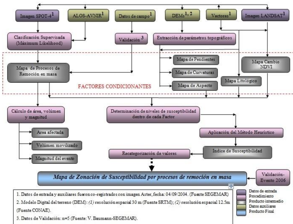
Figura 26. Representación esquemática que muestra los datos usados y procedimientos de trabajo realizados para la obtención del mapa de zonación de susceptibilidad por procesos de remoción en masa en la cuenca del río Tartagal. Ver texto para mayor detalle de cada paso.
