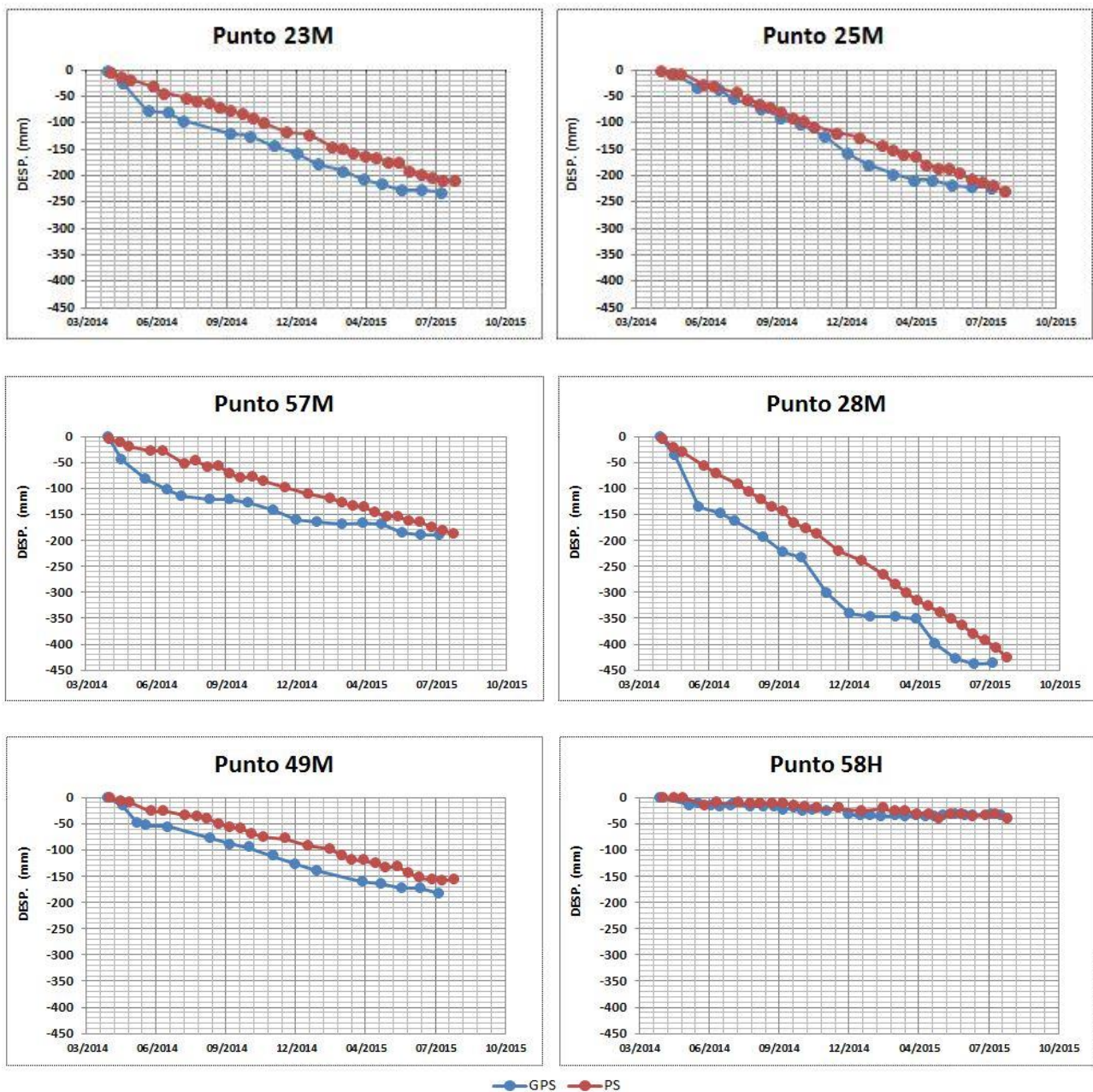
Figura 64: Comparación de series temporales de deformación para los puntos del área de alimentación.
