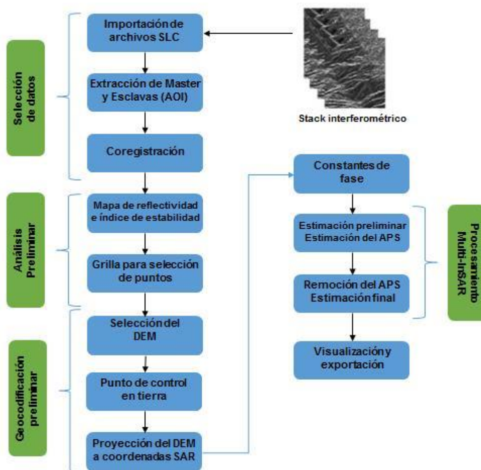
Figura 43: Flujo de trabajo PS convencional en SarProz (elaboración propia).
