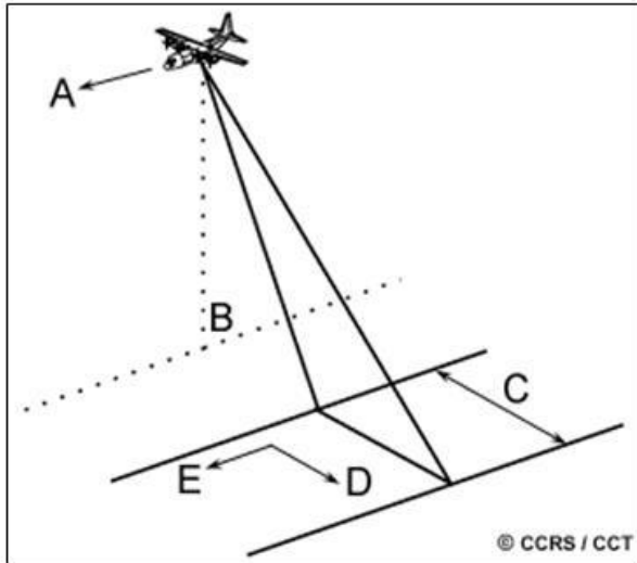
Figura 12: En la imagen de la izquierda, geometría de adquisición de un Radar, donde A indica la trayectoria de la plataforma, B indica el nadir, C indica el ancho de barrido o swath , D la dirección en rango y E la dirección en azimut. En la imagen de la derecha, A es el ángulo de incidencia local (en este caso del centro de la escena), B es el ángulo de mirada o Look Angle , C es el rango oblicuo o slant range , y D es el rango horizontal o ground range . (CCRS, 2006).
