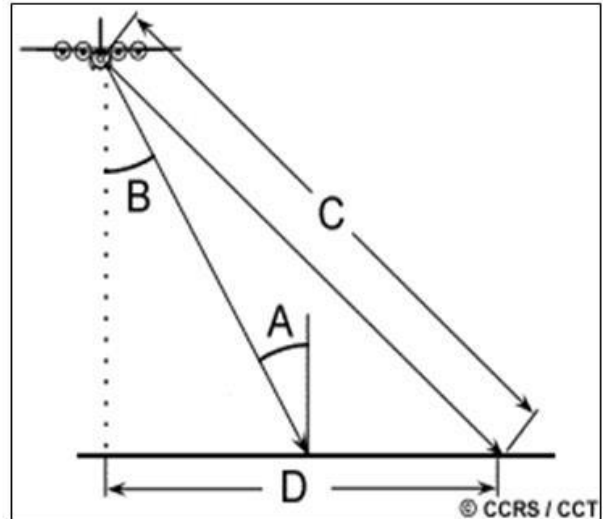
Figura 12: En la imagen de la izquierda, geometría de adquisición de un Radar, donde A indica la trayectoria de la plataforma, B indica el nadir, C indica el ancho de barrido o swath , D la dirección en rango y E la dirección en azimut. En la imagen de la derecha, A es el ángulo de incidencia local (en este caso del centro de la escena), B es el ángulo de mirada o Look Angle , C es el rango oblicuo o slant range , y D es el rango horizontal o ground range . (CCRS, 2006).
