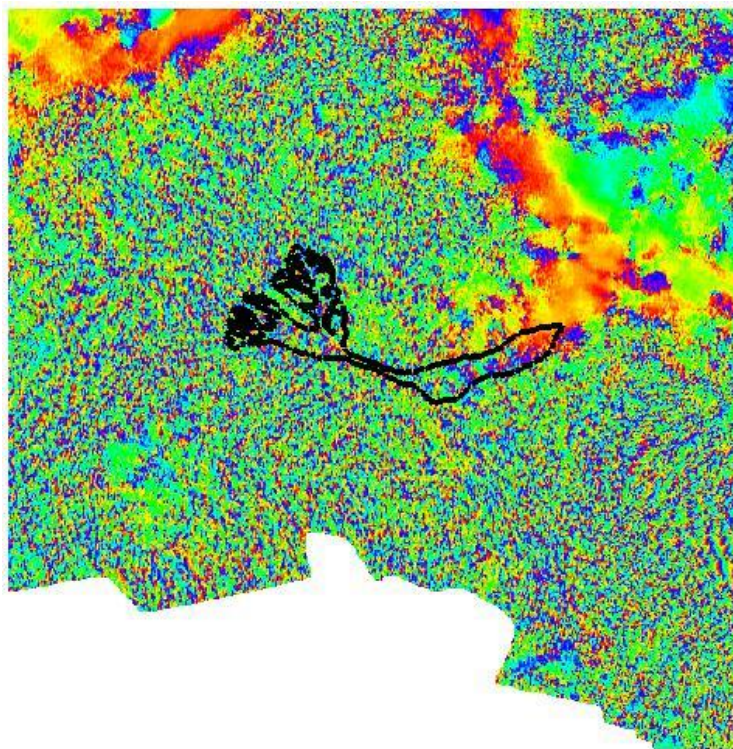
Figura 72: Interferograma diferencial para imágenes Sentinel-1A descendentes. B_{temp} = 24 días; B_N = 224.25 m. Coherencia media dentro del deslizamiento: 0,363. Fechas master/slave: 22-04-2015/04-05-2015.
