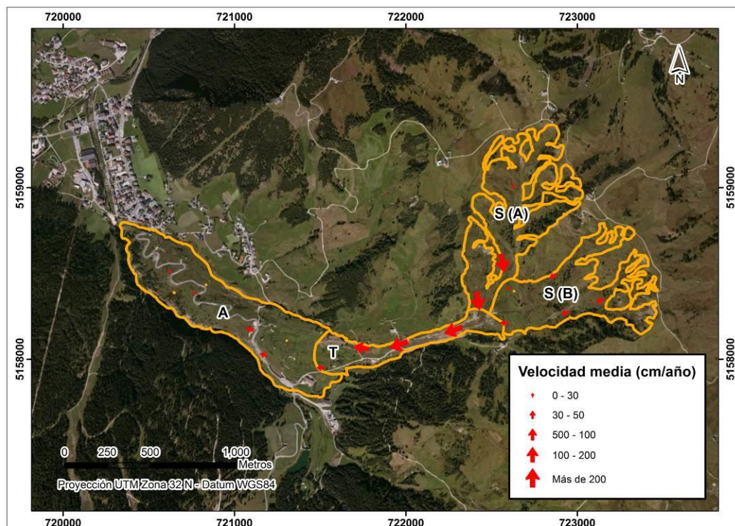
Figura 9: Velocidad y dirección de desplazamiento calculadas en las campañas GPS en el proyecto Corvara PSI Feasability. La zona de alimentación (A) se presenta como la más estable, la zona de transporte (T) es donde se registran la mayor cantidad de puntos veloces, y en la zona de alimentación se diferencia un sector más veloz S(A) de otro con velocidades más moderadas S (B) (Elaboración propia en base a datos provistos por EURAC Research).
