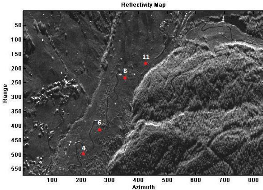
Figura 53: Mapa de reflectividad para la zona de acumulación en Slant Range. Corner Reflectors indicados con puntos rojos.
