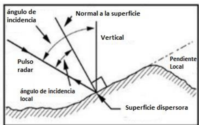
Figura 13: Con estas imágenes se busca graficar la diferencia entre el ángulo de incidencia y el ángulo de incidencia local. El primero se mide respecto a la normal al elipsoide, y siempre crece desde el rango cercano hacia el rango lejano. El segundo, en cambio, se mide respecto a la normal a la pendiente local, y su variación puede no ser tan constante. En terrenos planos, ambos ángulos tenderán a coincidir. Fuente: (CCRS, 2006)
