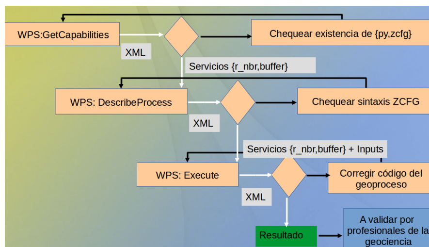
Figura 5.6: Procedimiento para testear los servicios web de procesamiento.
