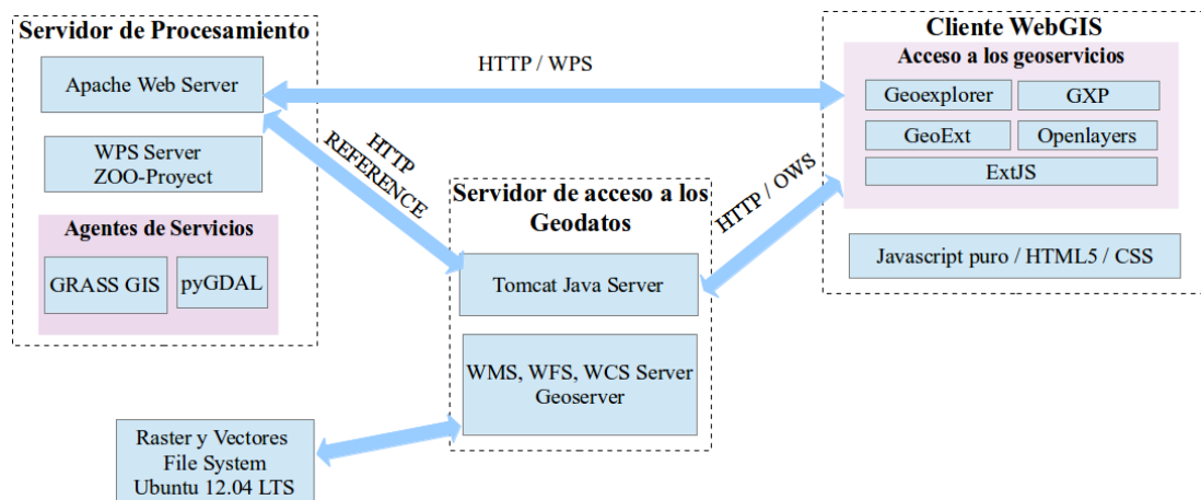
Figura 4.8: Arquitectura con las tecnologías elegidas
