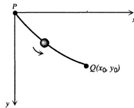
Figura 2: La braquistócrona.
